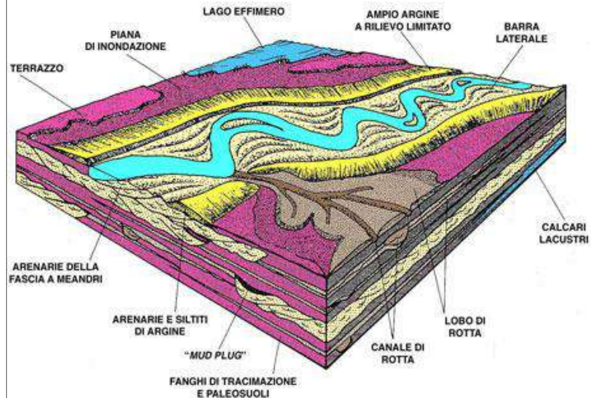
ELEMENTI ARCHITETTURALI DEL CONTESTO DI TRACIMAZIONE (da Miall, 1996)
