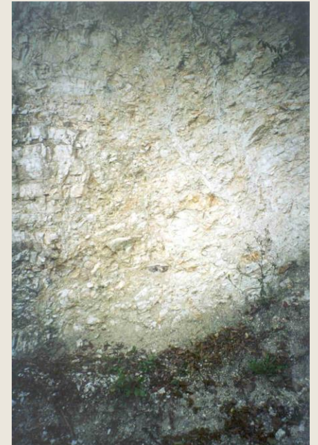
(Foglio 49, Verona, Carta Geologica d'Italia échelle 1:100.000, Modifiée)
