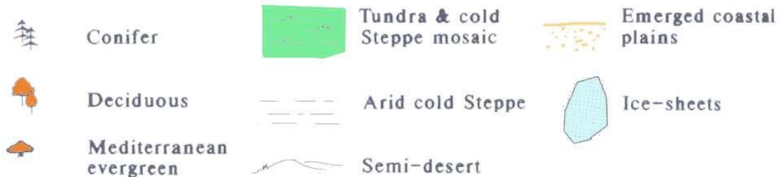
MIS 6, circa 150.000 anni fa (d'après Van Andel 1996)
