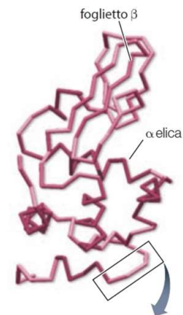
(B) Modello a bastoncini
