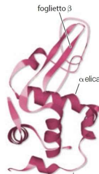
(C) Modello a nastro
