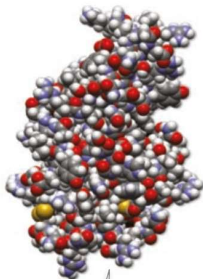
(A) Modello a spazio pieno
