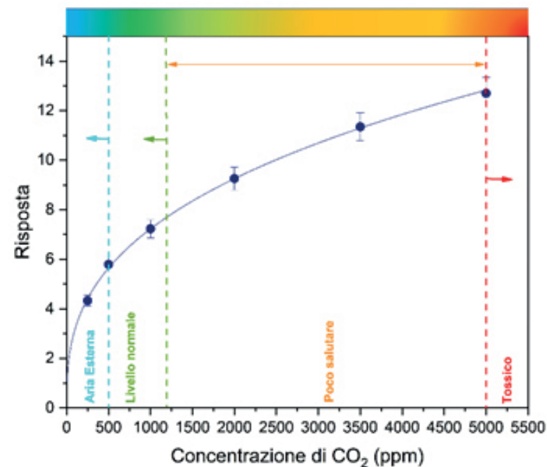
(Curva di calibrazione ottenuta esponendo il film sensibile a diverse concentrazioni di CO 2 )
