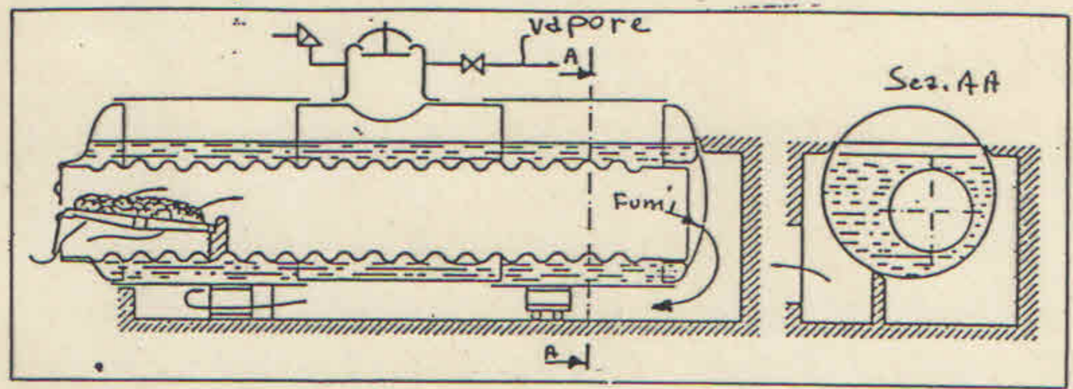
CALDAIA CORNOVAGLIA
