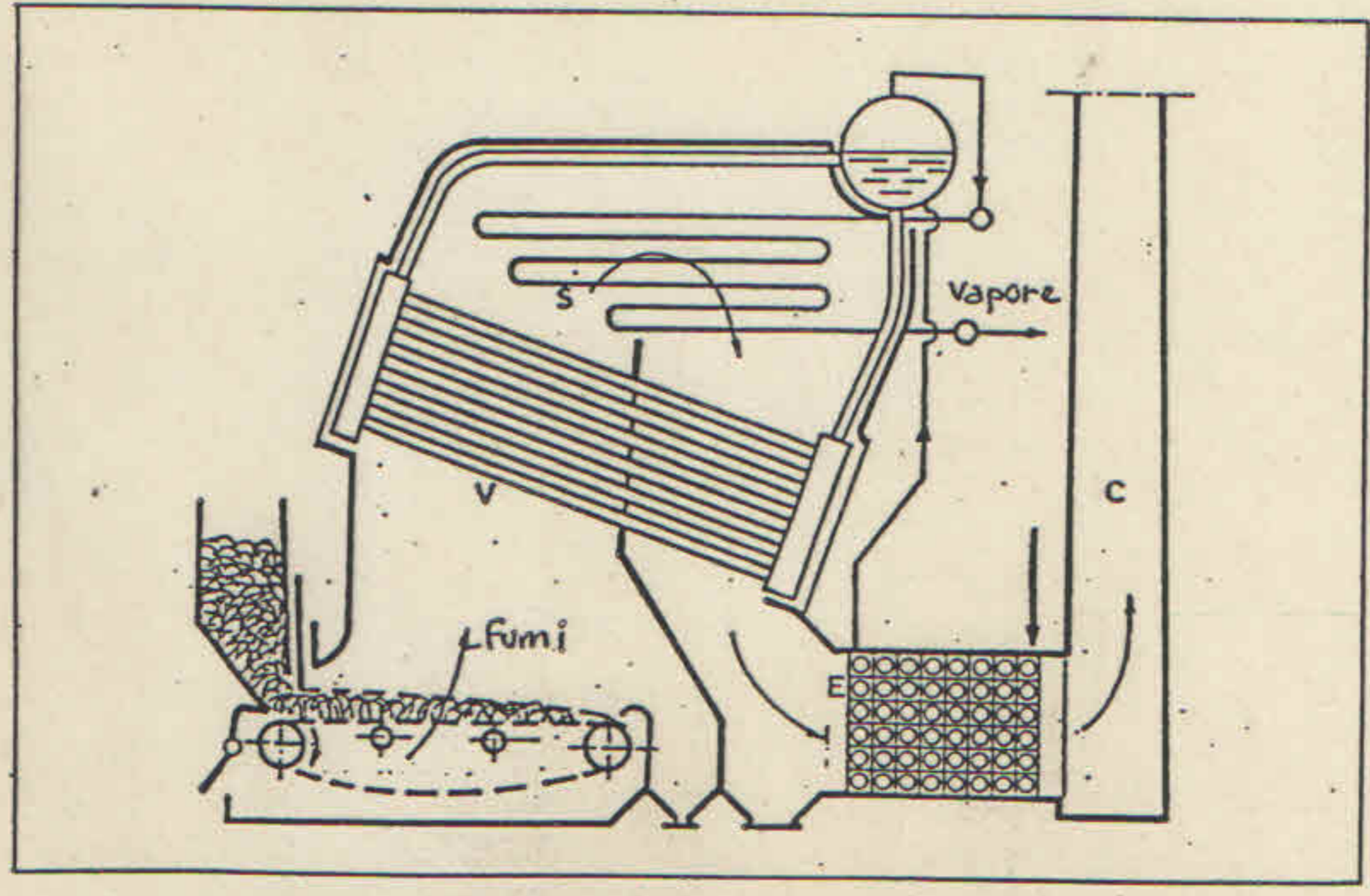
CALDAIA BABCOK
