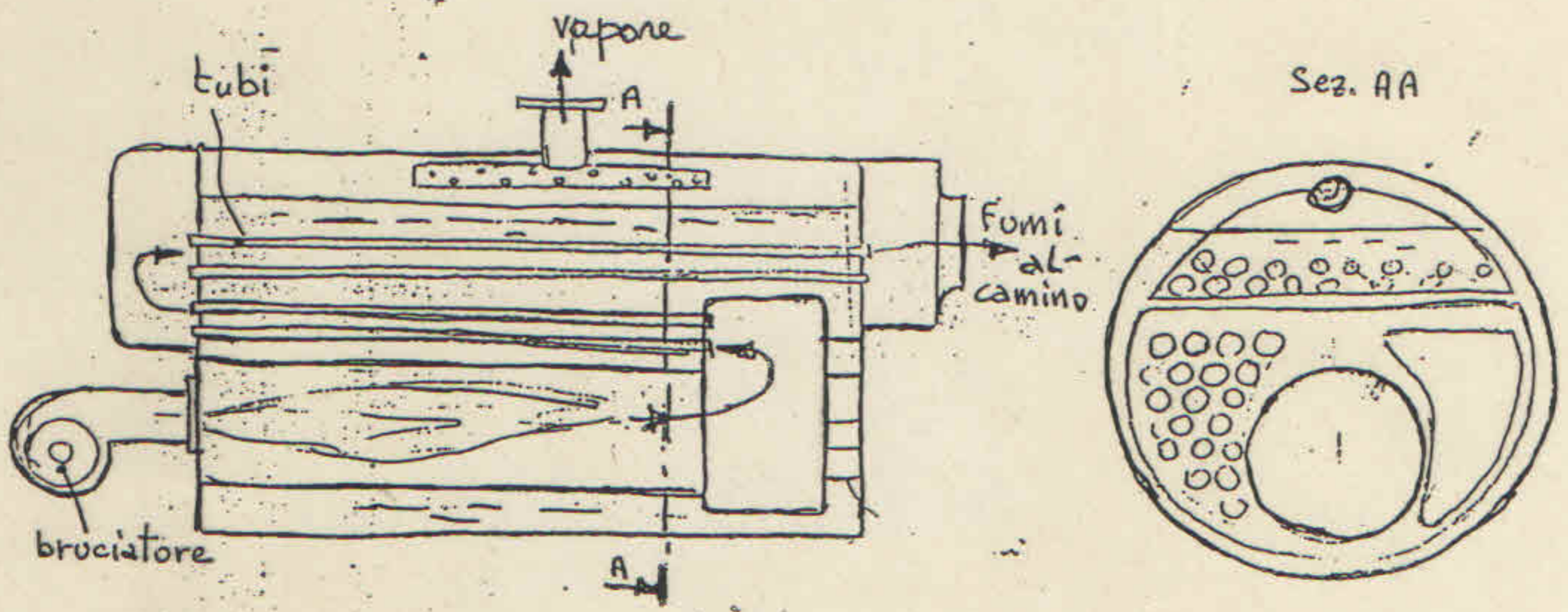
CALDAIA MARINA
