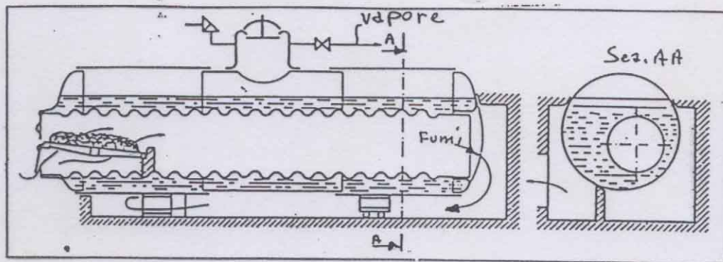
CALDAIA CORNOVAGLIA
