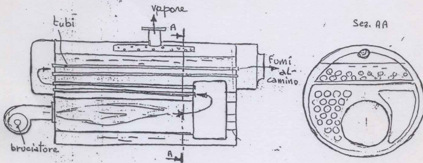
CALDAIA MARINA
