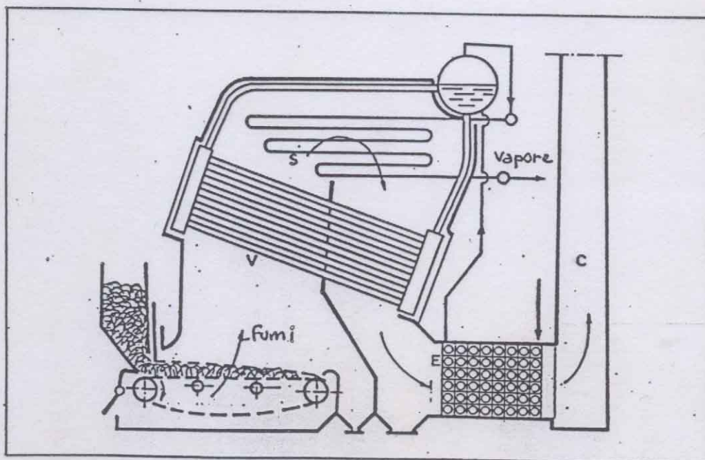
CALDAIA BABCOK
