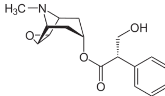
SCOPOLAMINA
