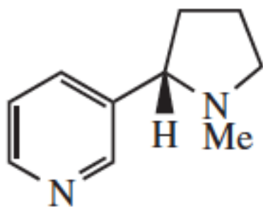
nicotine
