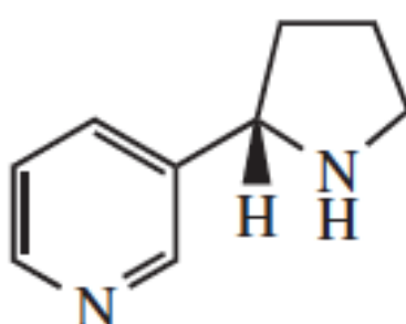
nornicotine
