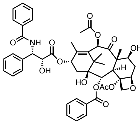
TASSOLO (PACLITAXEL)
