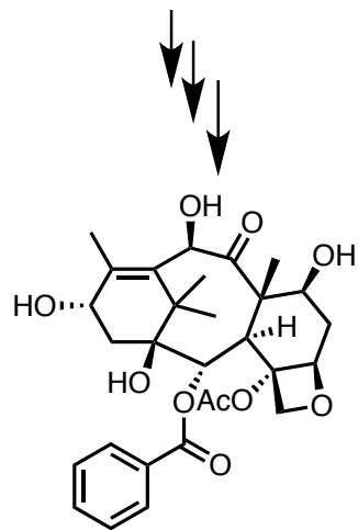
10-Deacetylpaclitaxina III
