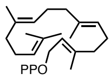
Geranylgeranylpirofosfato
