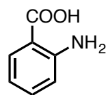
Ac. Antranilico
