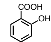
Ac Salilico
