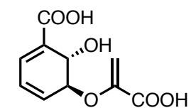
Ac Isocorismico
