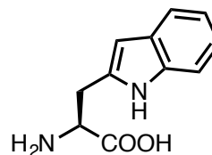
L-Triptofano
