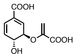
Ac Corismico
