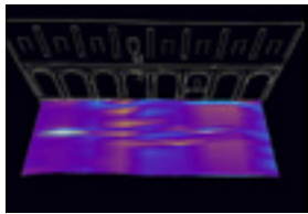
Chiesa di S. Salvatore al Monte, Firenze visualizzazione della deformazione del pavimento sulla base del modello 3D derivante dal modello topografico Università di Firenze, Istituto Geografico Militare Church of S. Salvatore al Monte in Florence visualization of the floor deformation on the basis of a 3D model generated from topographic survey
