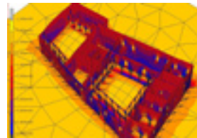
Casa Romei, Ferrara Esempio di analisi FEM Soprintendenza di Ravenna
