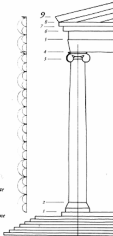
rappresentazione schematica dell'ordine ionico ellenistico
