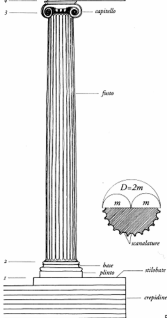
Magnesia al Meandro (Ionica) tempio di Artemis Leucophriene (fine del III secolo a.C.)
