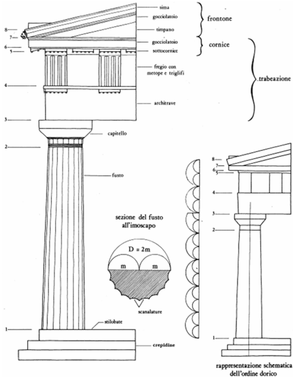
OLIMPIA ( 468-460 a.C.) Tempio di Zeus
