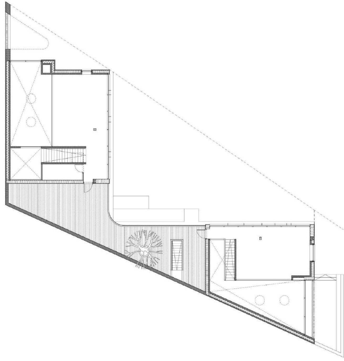
DDS, Plan 1. Mål 1:200
