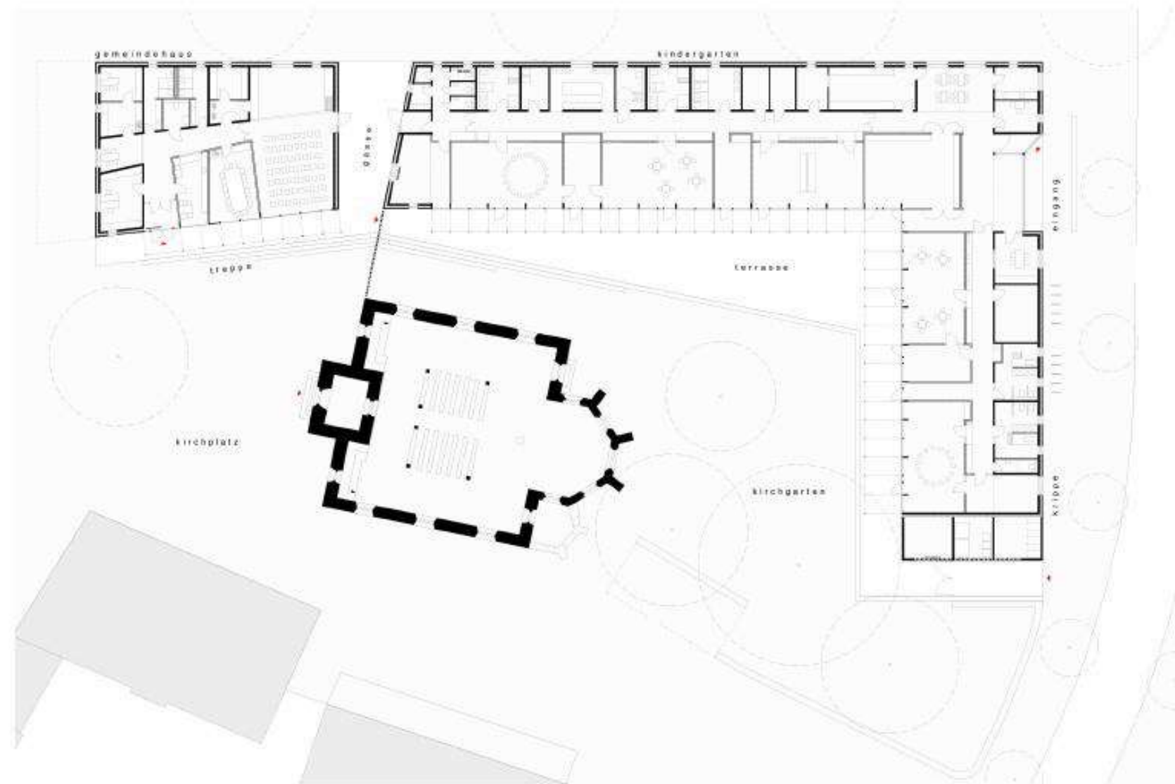
gemeindezentrum st. marien | hannover hainholz grundriss 1:500
