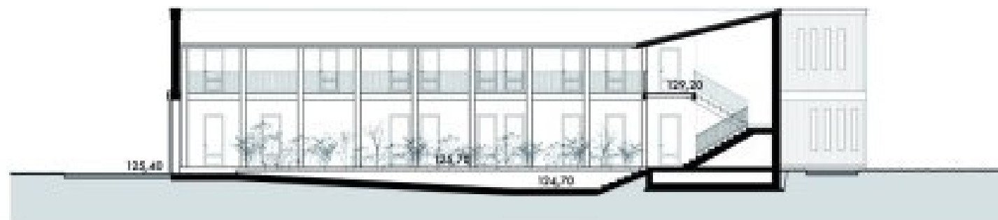
SEZIONE B-B
