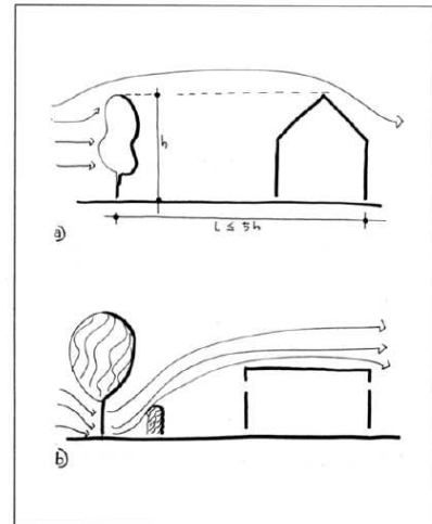
Figura 2.42. a) Effetto schermante da essenza vegetale con chioma compatta; b) effetto frangivento da essenza vegetale con l'utilizzo di siepi protettive.
